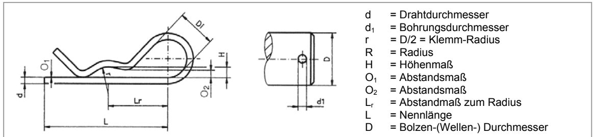
Abbildung: Schematische Darstellung Federstecker
